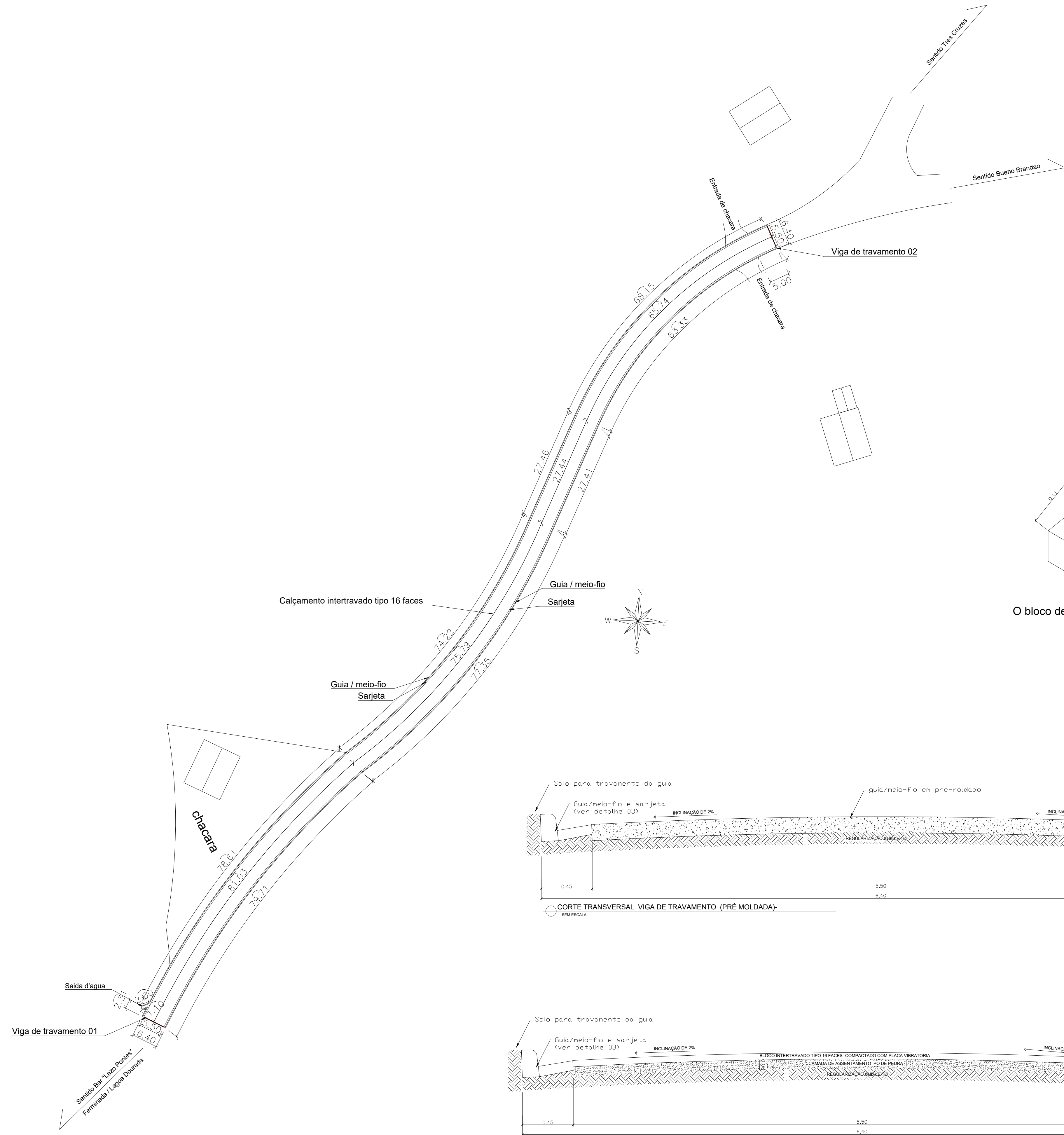
PLANTA CALÇAMENTO SEM ESCALA
