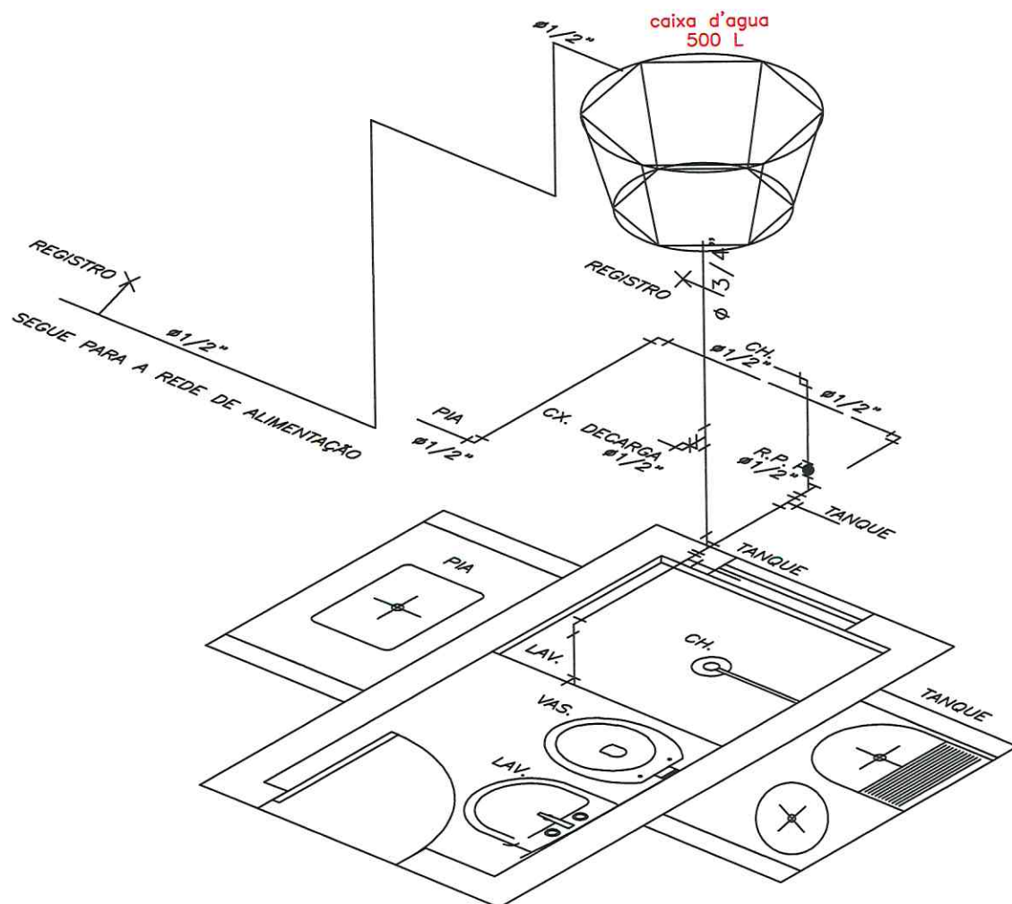
ISOMÉTRICO — HIDRÁULICA ESC. 1/20
