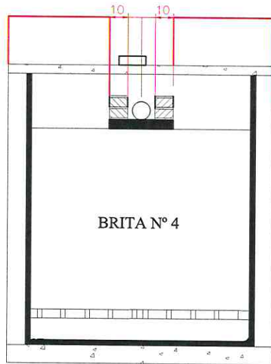
CORTE GG
